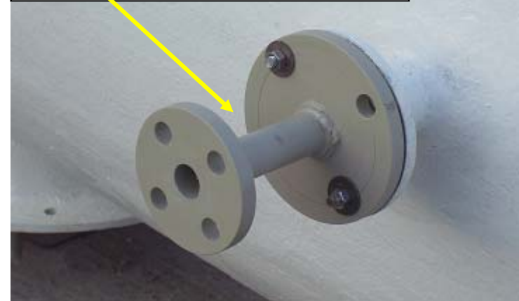
Boquillas flangeadas en polipropileno para sistema aspersión
