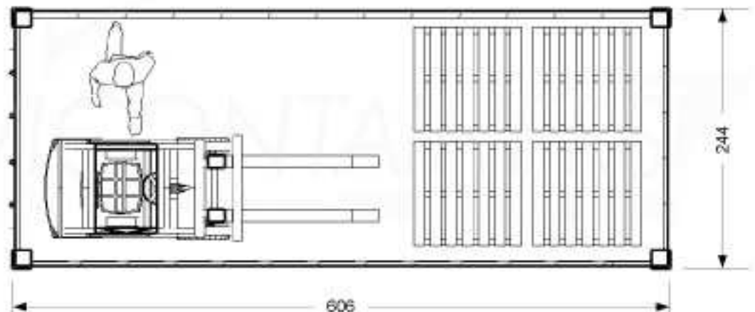
Vista Planta
